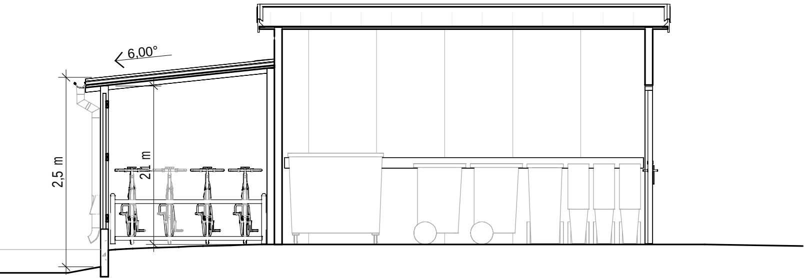
SEKTION 1
