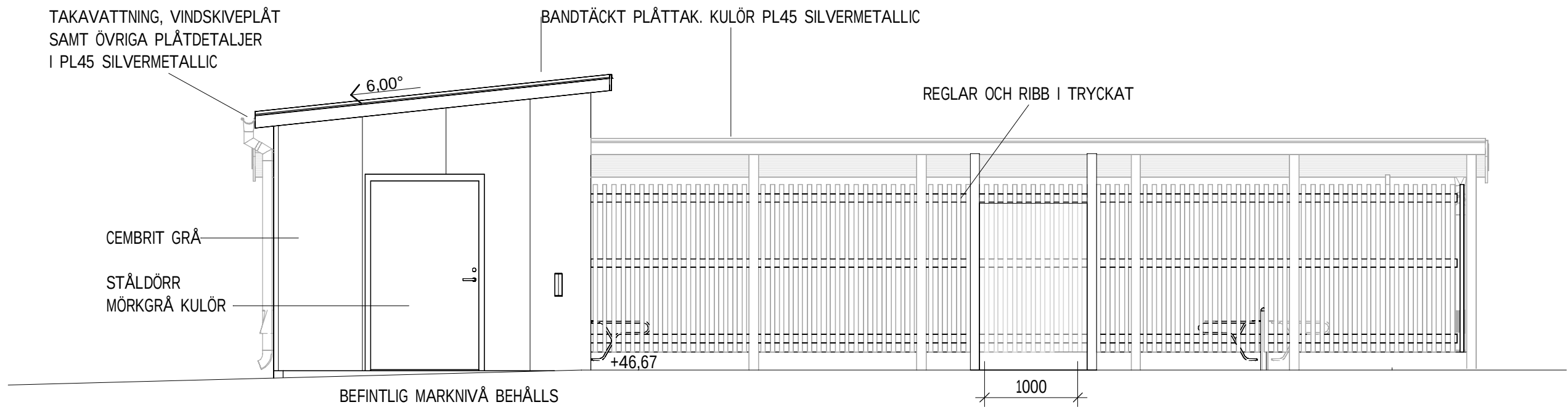
AVFALLSRUM - FASAD MOT NORDOST, PARKERING
