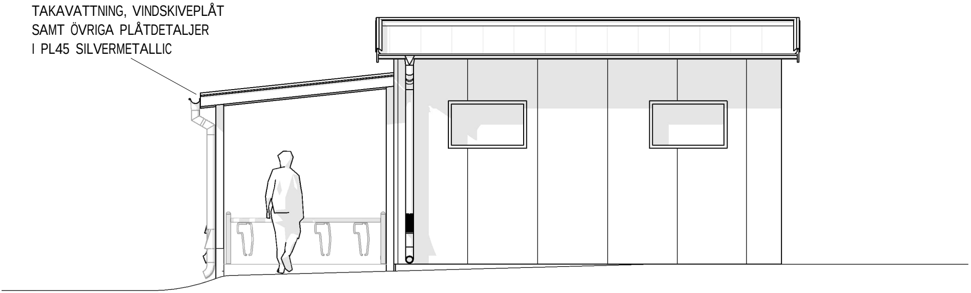
AVFALLSRUM - FASAD MOT SYDOST, ROSENIEGATAN
