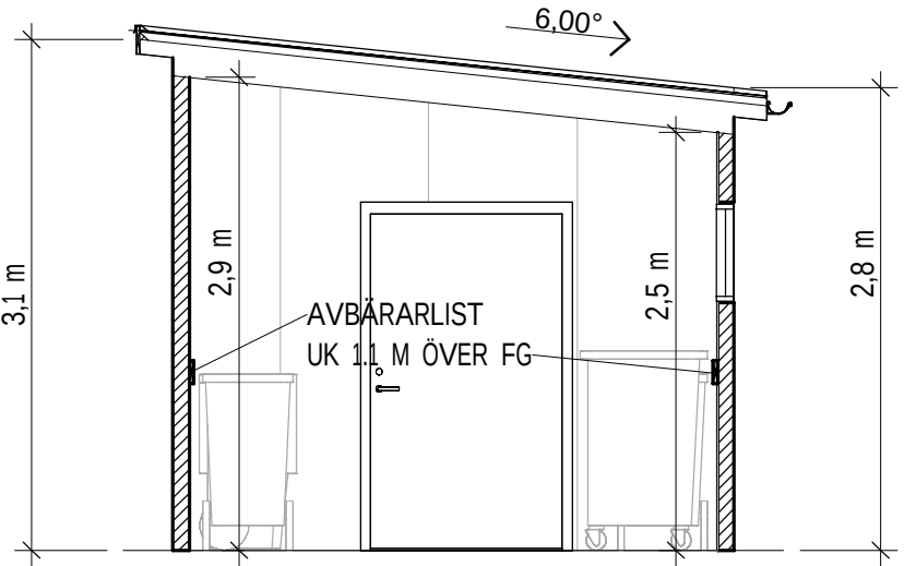
SEKTION 2
