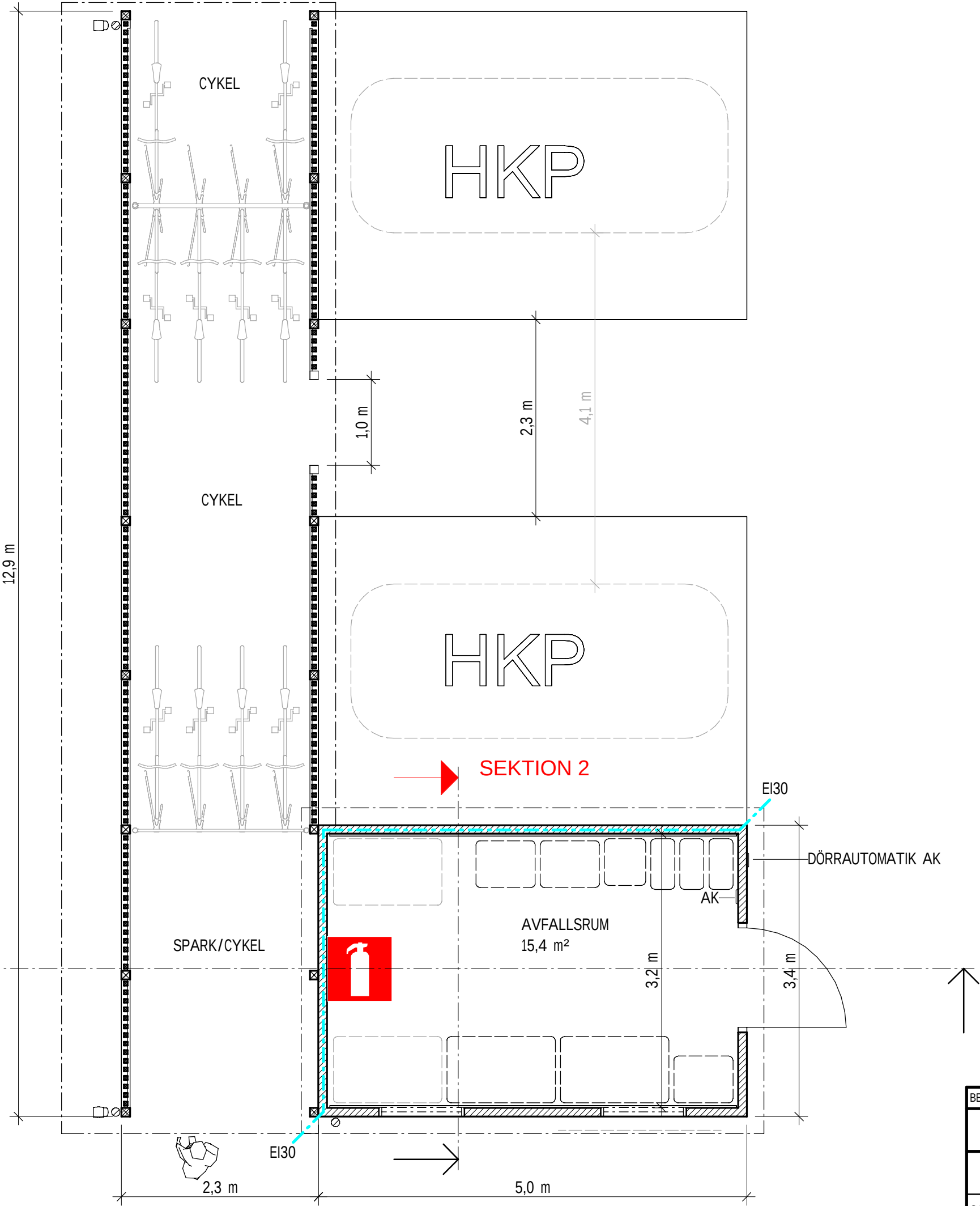
AVFALLSRUM - PLAN
